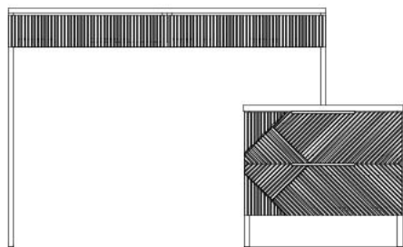
Исполнение 1
